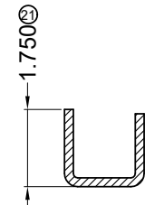
SECTION D-D SCALE 1:1
